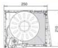
VEKAVARIANT 210 mm Revision vorne mit Insektenschutz
