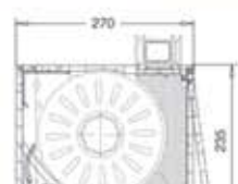
VEKAVARIANT 235 mm Revision vorne mit Insektenschutz
